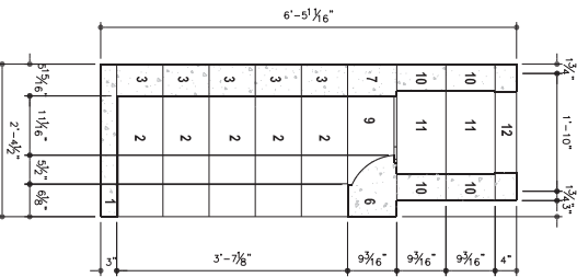
SECTION A-A SCALE: 1" = 1'-0"
