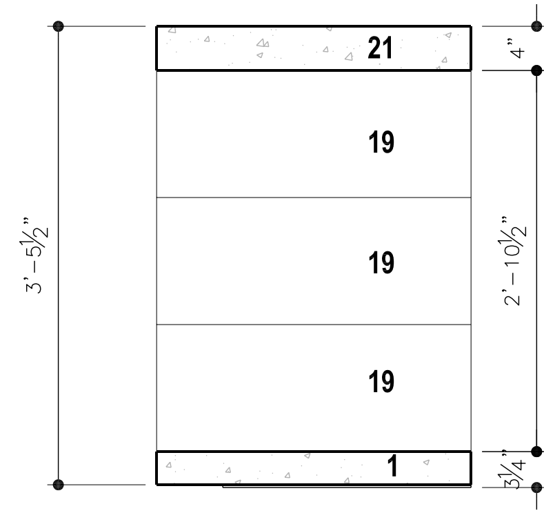
SECTION A-A - ALT
